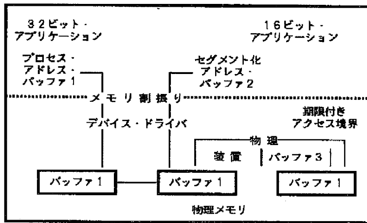
メモリ割振り方式のアプリケーション例
